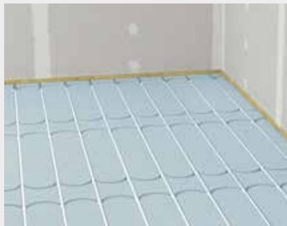
Instalace trubek podlahového vytápění 16 mm
